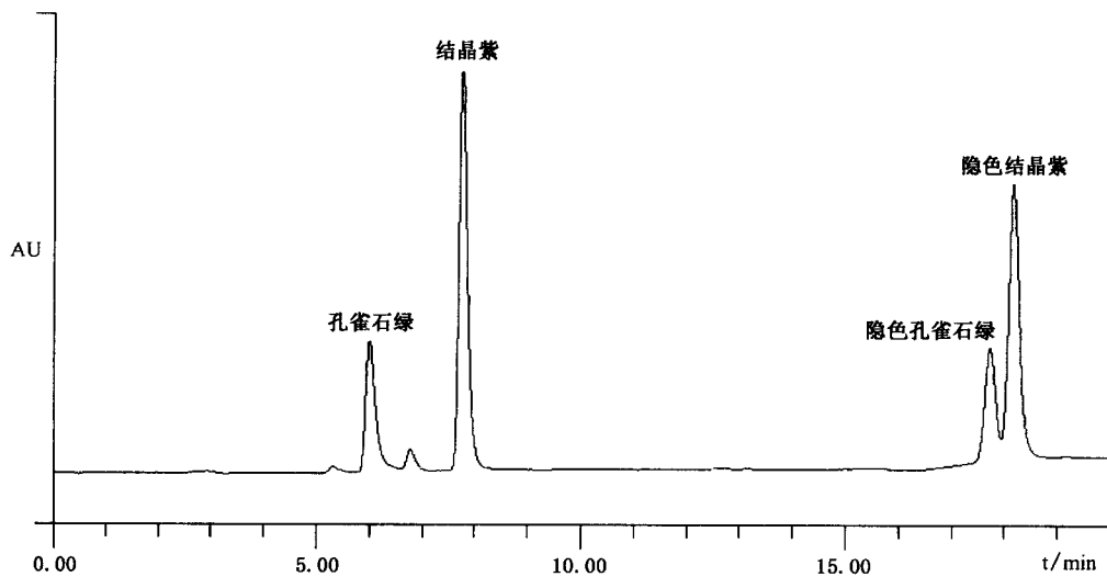
图 A.1 孔雀石绿、隐色孔雀石绿、结晶紫、隐色结晶紫、氘代孔雀石绿和氘代隐色孔雀石绿标准的离子流图
